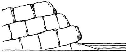
चित्र १३३—कगार का खनन (तहों का नमन समुद्र के विपरीत ओर)।
